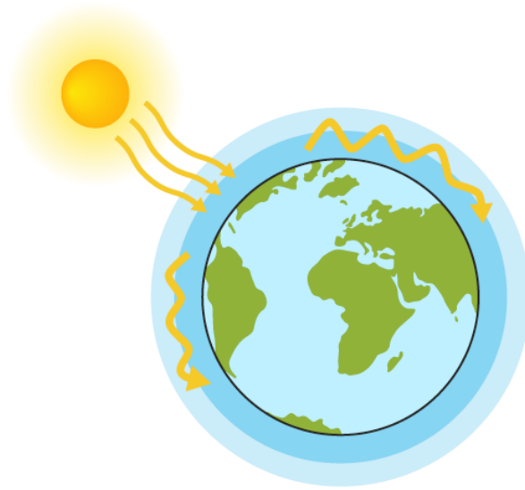
Formation de la couche d'ozone
